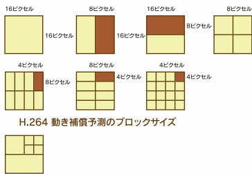
H.264 動き補償ブロックのパターン
